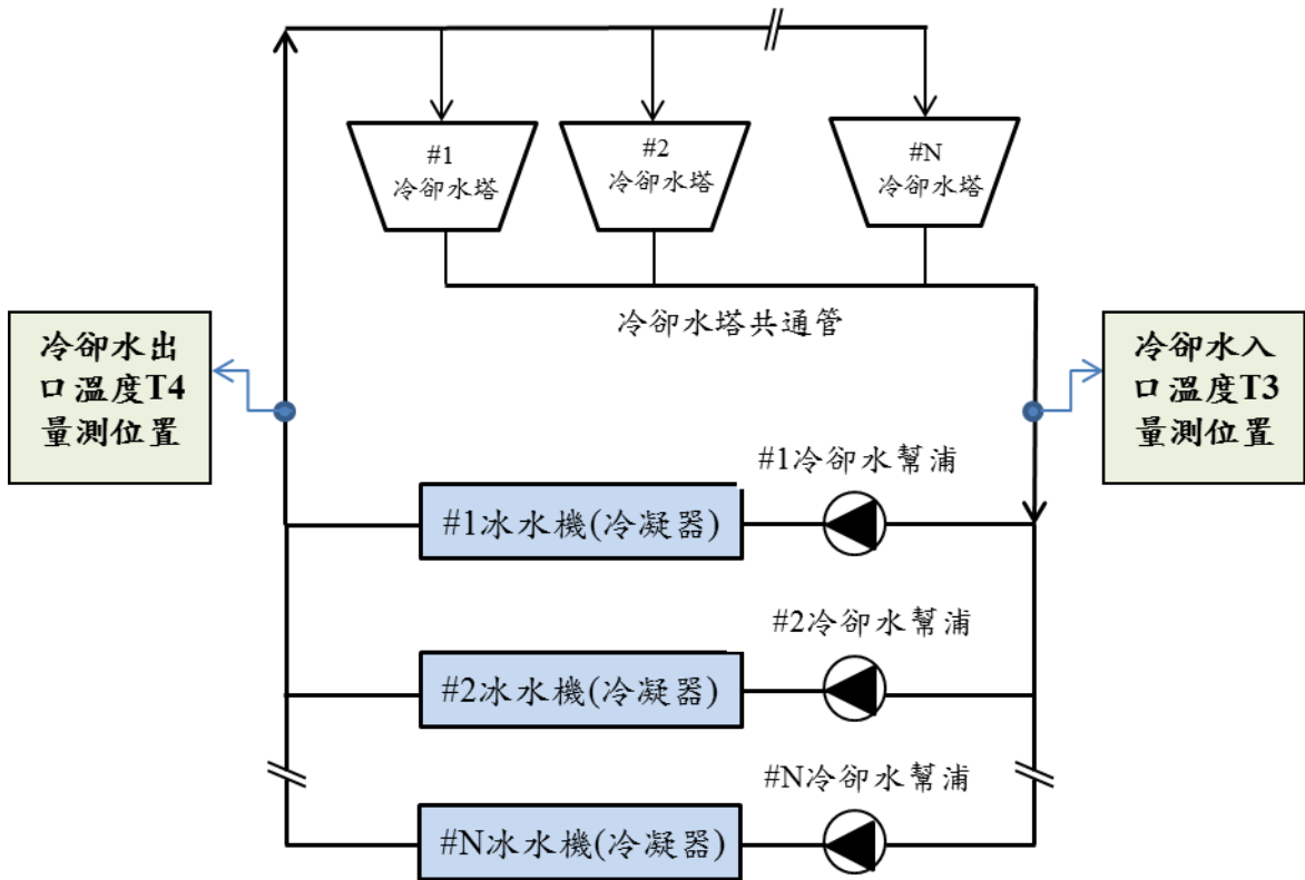
圖四 冰水機冷凝器冷卻水出水、回水溫度差量測位置
