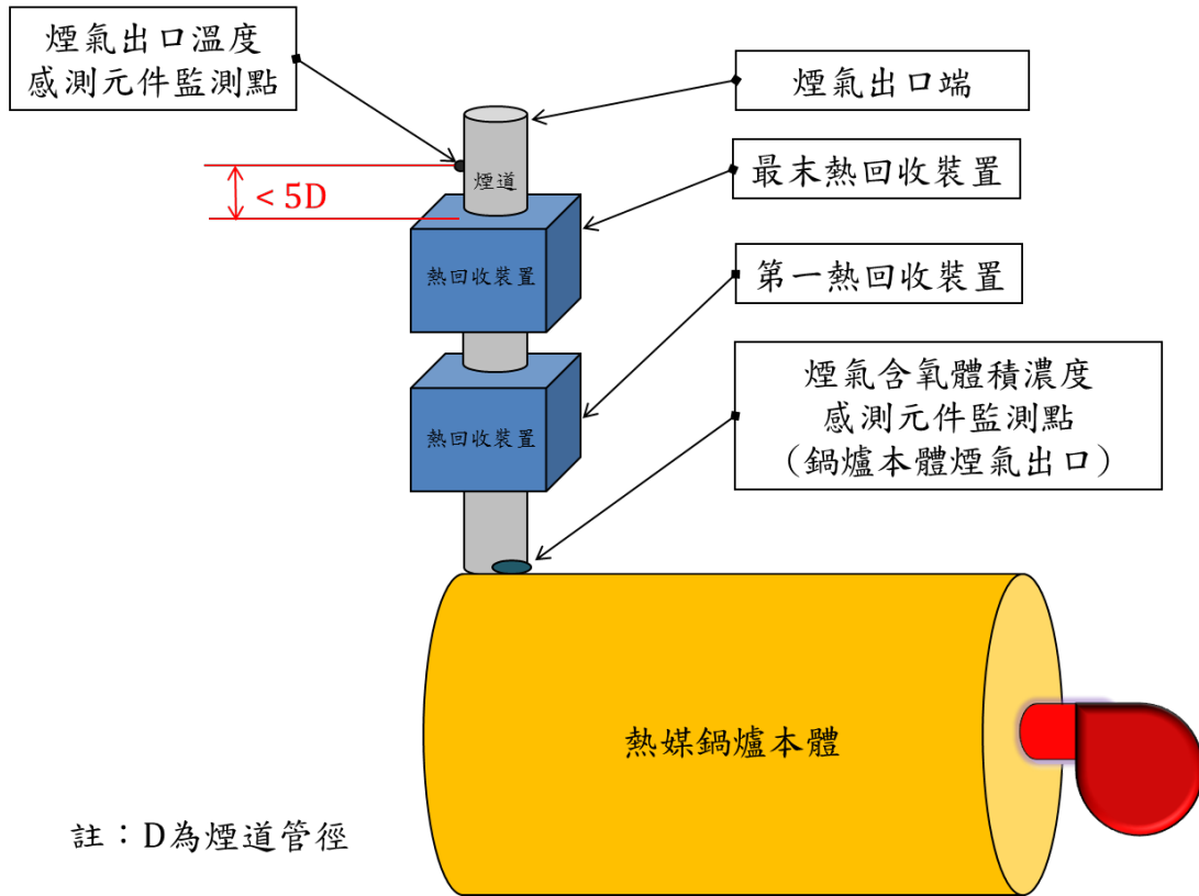
圖四 熱媒鍋爐（已設置熱回收裝置）煙氣含氧體積濃度及煙氣出口溫度之監測點
