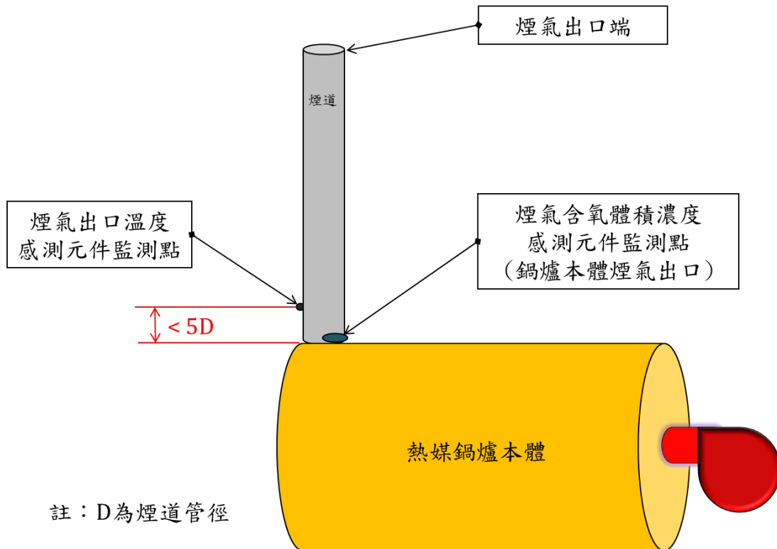
圖三 熱媒鍋爐（未設置熱回收裝置）煙氣含氧體積濃度及煙氣出口溫度之監測點
