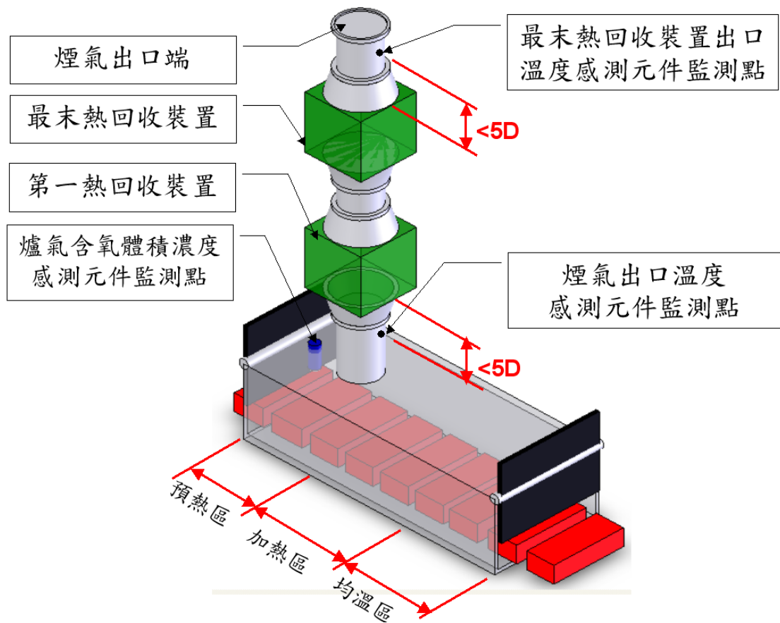
圖二 連續式加熱爐（設有熱回收裝置）爐氣含氧體積濃度感測元件及溫度感測元件設置點示例
