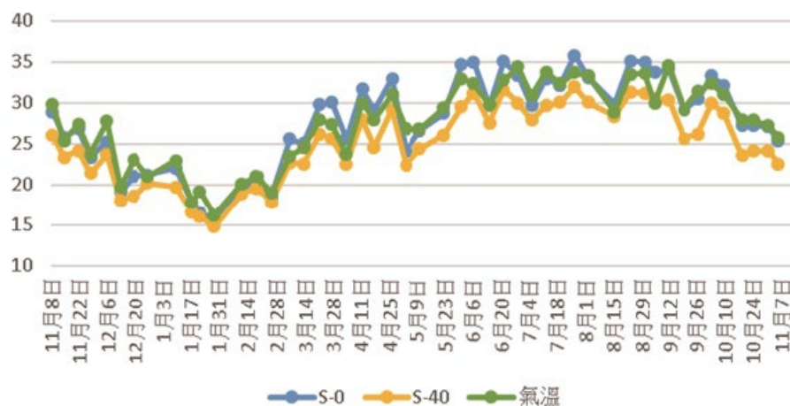
圖 2-14：池水水溫折線比較圖
