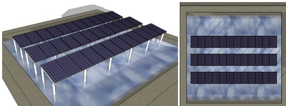
圖 2-6：立柱型示意圖(含俯視圖)
