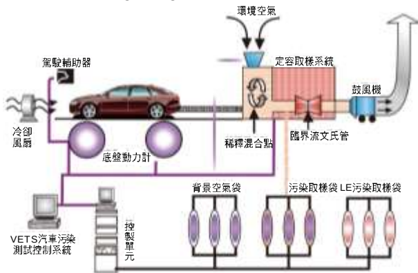
車輛能源效率及污染測試實驗室相關設備示意圖
